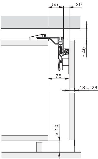
外盖门, 不带底部型材
