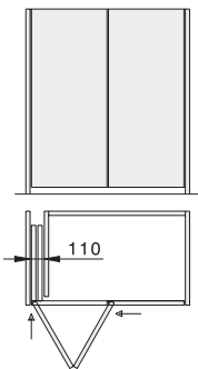
外盖门, 不带底部型材
