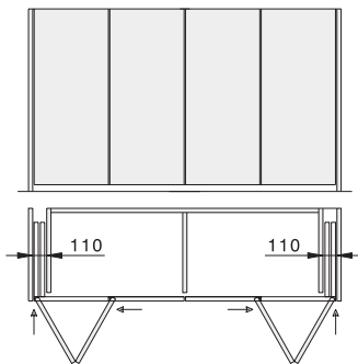
一门到顶无底板
